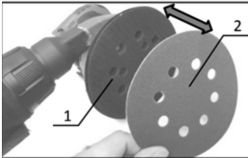
1. Base de fixação da lixa 2. Lixa
